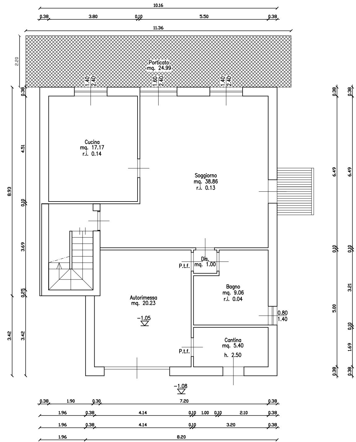
PIANO TERRENO H. 2.70 CORPO DI FABBRICA 2
