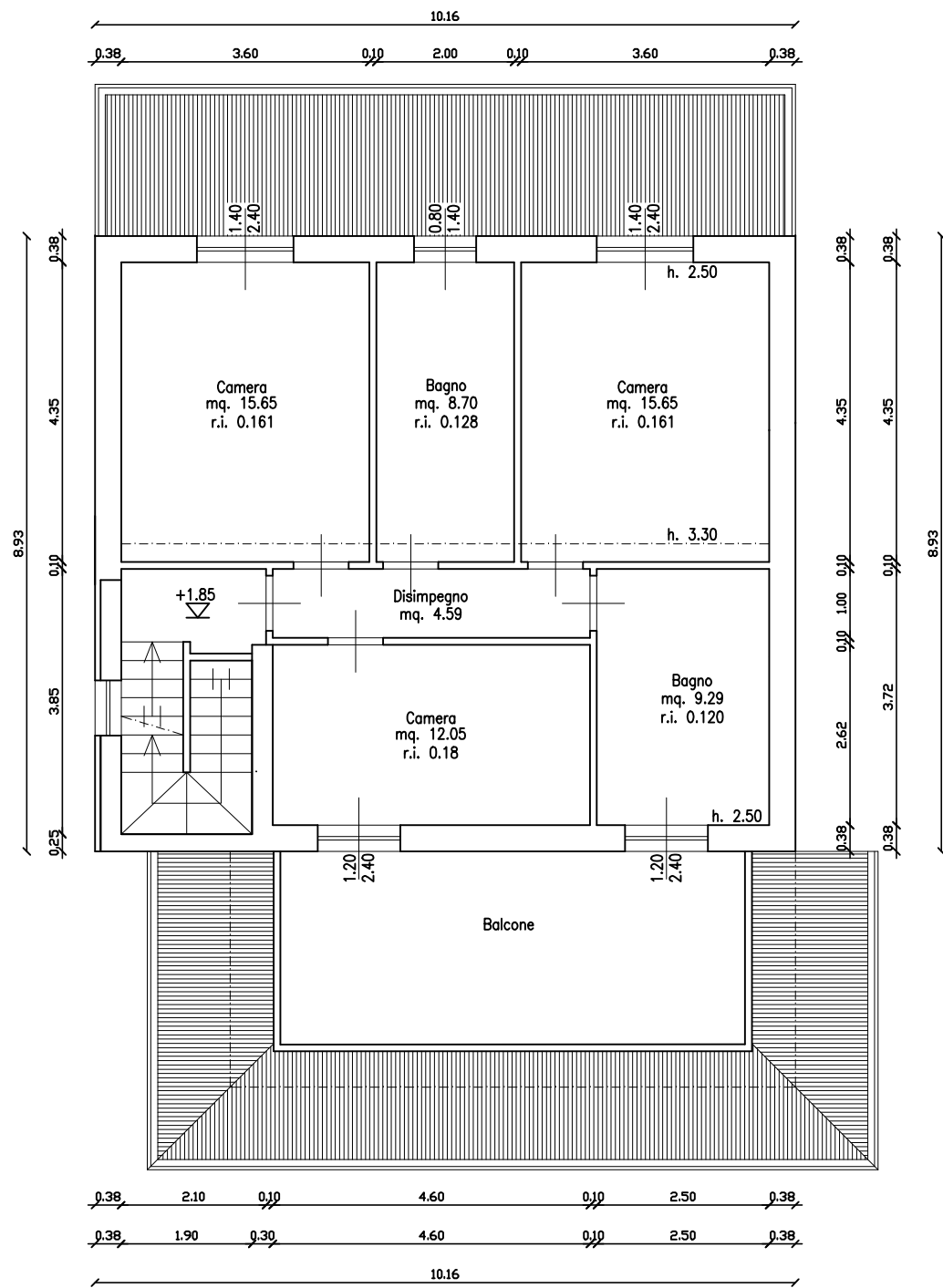
PIANO PRIMO CORPO DI FABBRICA 2
